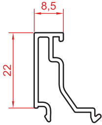
1948 0.239 kg/m
