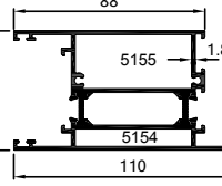
55-4300-4302 2.163 kg/m
