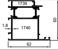
55-1700-1716 1.377 kg/m
