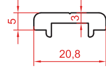
1755 0.234 kg/m
