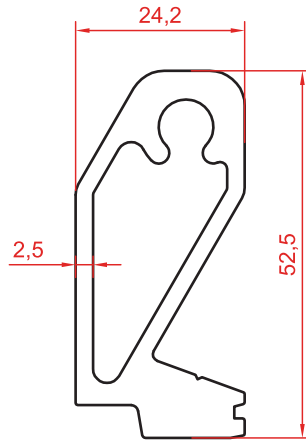
1766 1.352 kg/m
