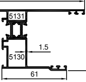
55-5130-5131 1.619 kg/m
