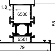
55-1704-1717 1.615 kg/m
