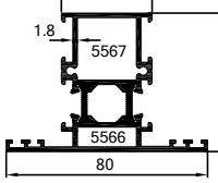
55-1650-1651 1.811 kg/m
