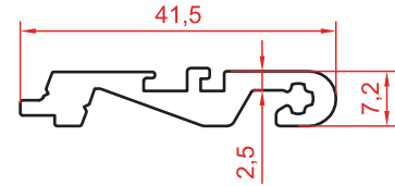
1774 0.480 kg/m
