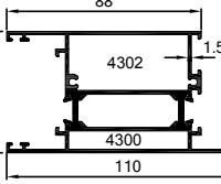
55-5525-5526 2.140 kg/m
